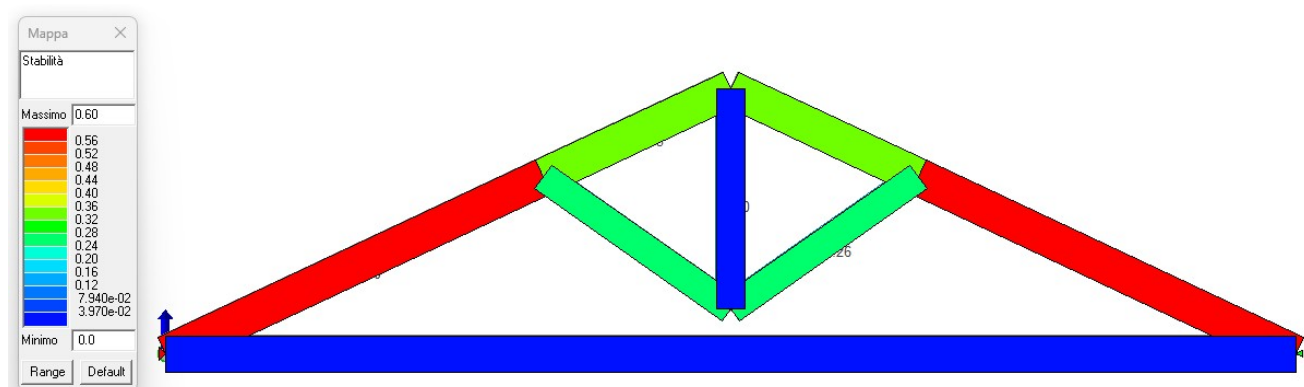
Figura 19. Verifica a stabilità agli SLU
