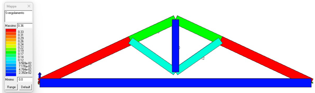
Figura 20. Verifica a svergolamento agli SLU
