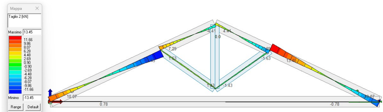
Figura 13. Sollecitazioni di taglio agli SLU
