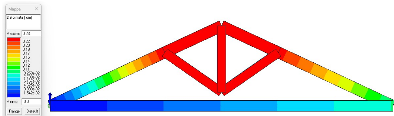
Figura 21. Deformata massima agli SLU
