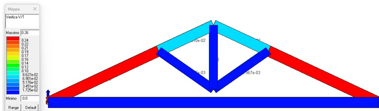
Figura 18. Verifica a taglio-torsione agli SLU
