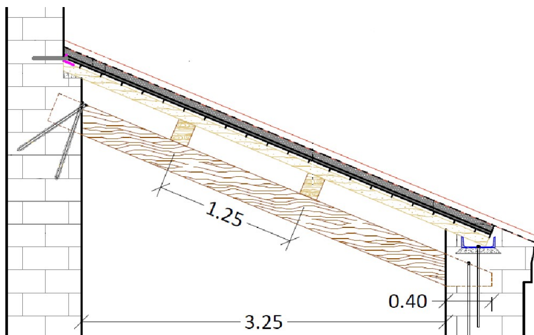
Figura 6. Progetto strutturale navata laterale
