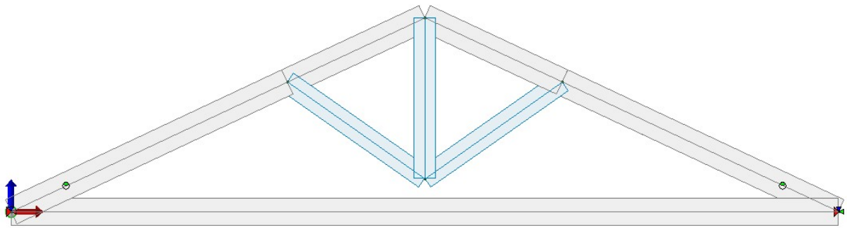
Figura 11. Modello 3D agli elementi finiti della capriata
