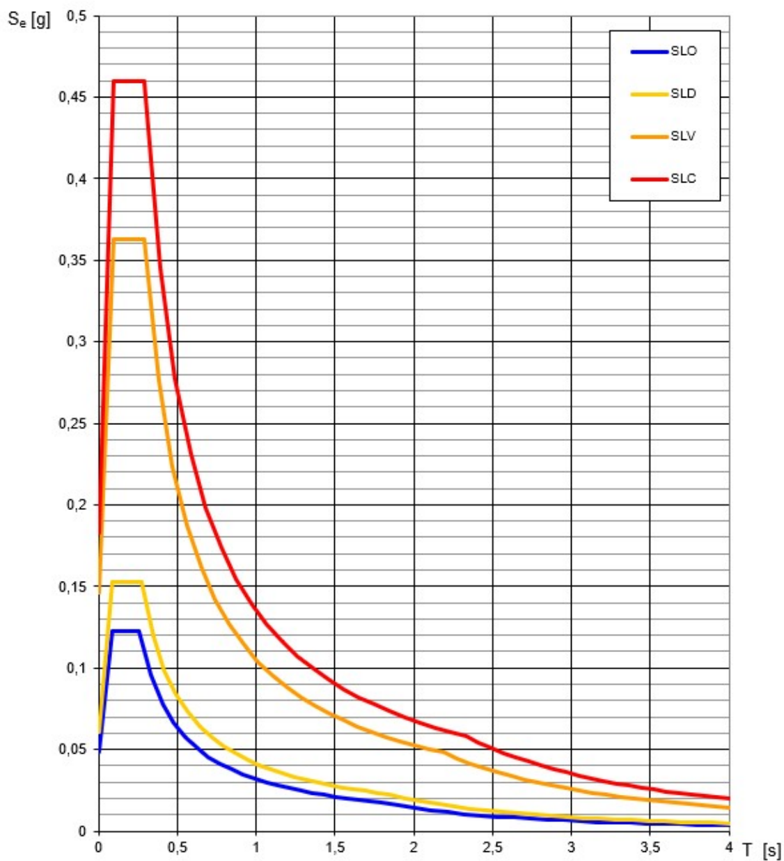
Figura 9. Spettri di progetto
