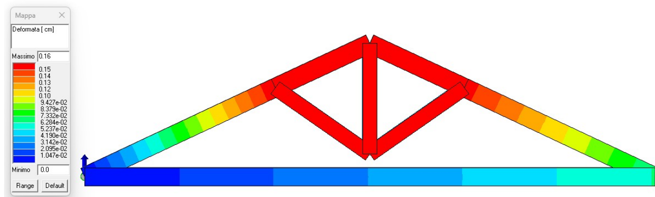
Figura 23. Deformata massima agli SLE
