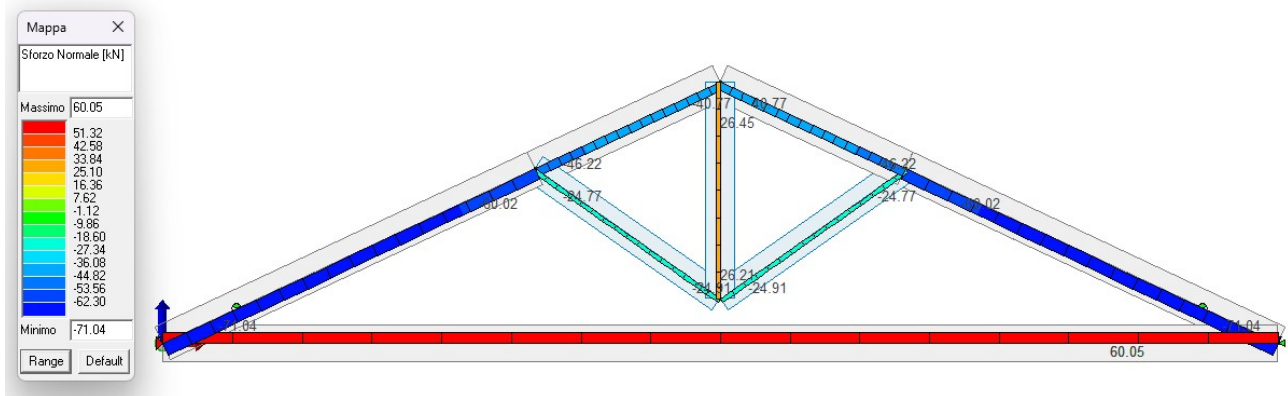
Figura 12. Sforzo Normale agli SLU
