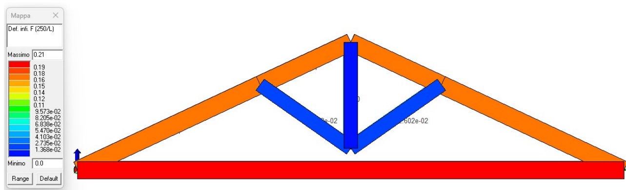
Figura 22. Verifica agli SLE
